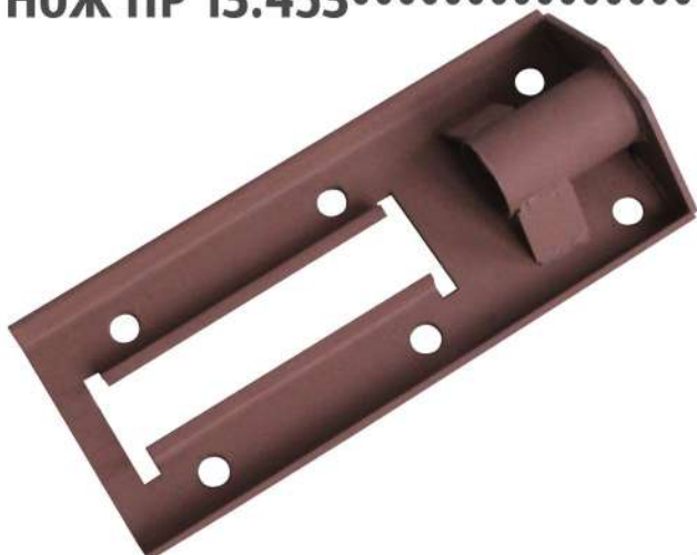
Основание ПР-1,4.52.08.000 (натяжного устройства)••
